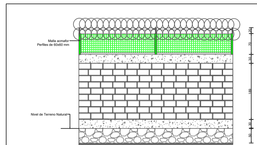
MURO CORRESPONDIENTE A 25 METROS LINEALES - SECTOR: FRENTE A MULTICANCHA - INSTALACIÓN DE MALLA ACMAFOR - INSTALACIÓN DE CONCERTINA DOBLE
