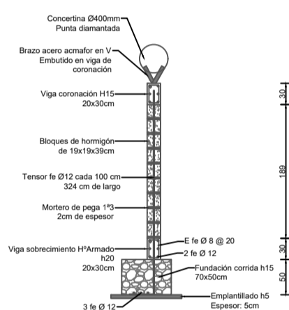
MURO CON BLOQUES DE HORMIGÓN - 27,5 METROS LINEALES - INSTALACIÓN DE CONCERTINA
