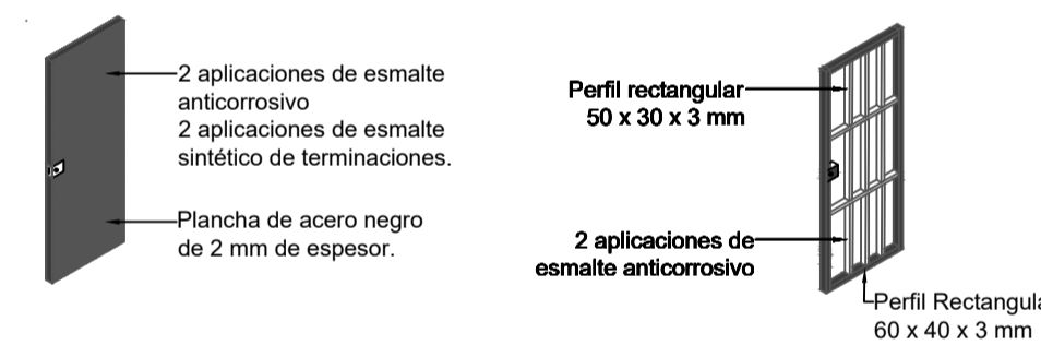
DETALLE PUERTA DE SEGURIDAD
