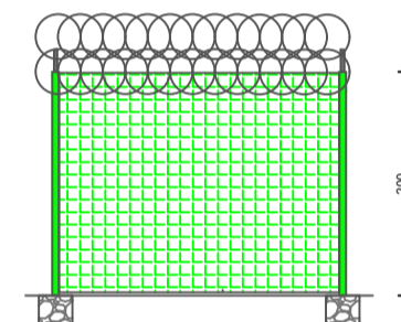
- 285 METROS MALLA ACMAFOR - CONCERTINA DOBLE
